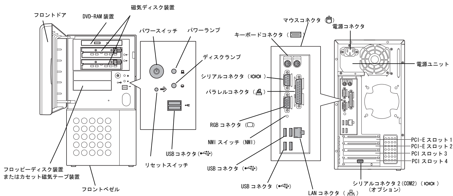
正面図（フロントドアが開いた状態）
