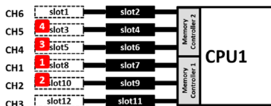
実装されるメモリが 4 枚の場合
