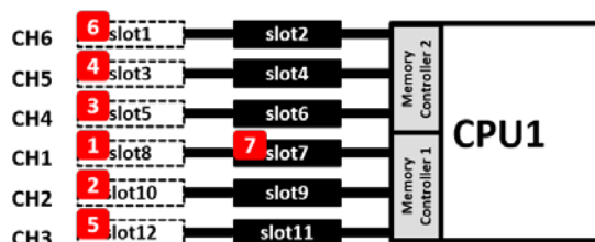
実装されるメモリが 5～7 枚の場合
