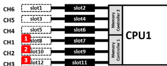
実装されるメモリが 1～3 枚の場合
