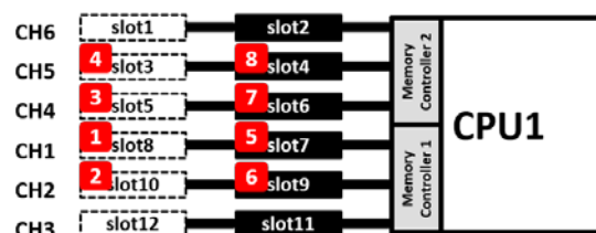
実装されるメモリが 8 枚の場合
