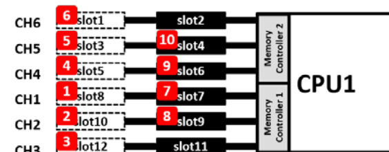
実装されるメモリが 10 枚の場合
