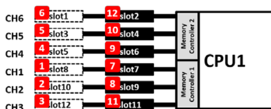
実装されるメモリが 11～12 枚の場合
